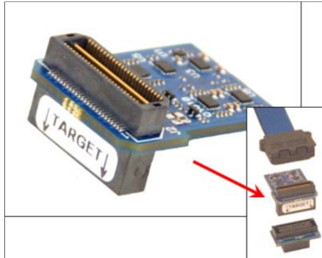
MIPI-60/34 Mini Cable Adapter for XDS560v2
