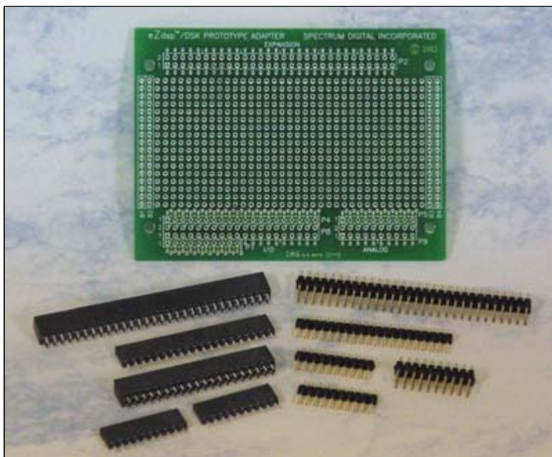
Wire Wrap Prototyping Module for eZdsp
